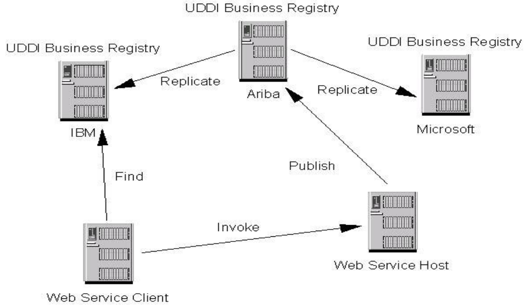
Şekil 5.7 – UDDI Kurum Kayıt Sunucuları (Kaynak numarası : 63)
