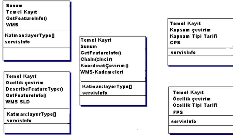
Şekil 2.13 Haritacılık sınıf diyagramları
