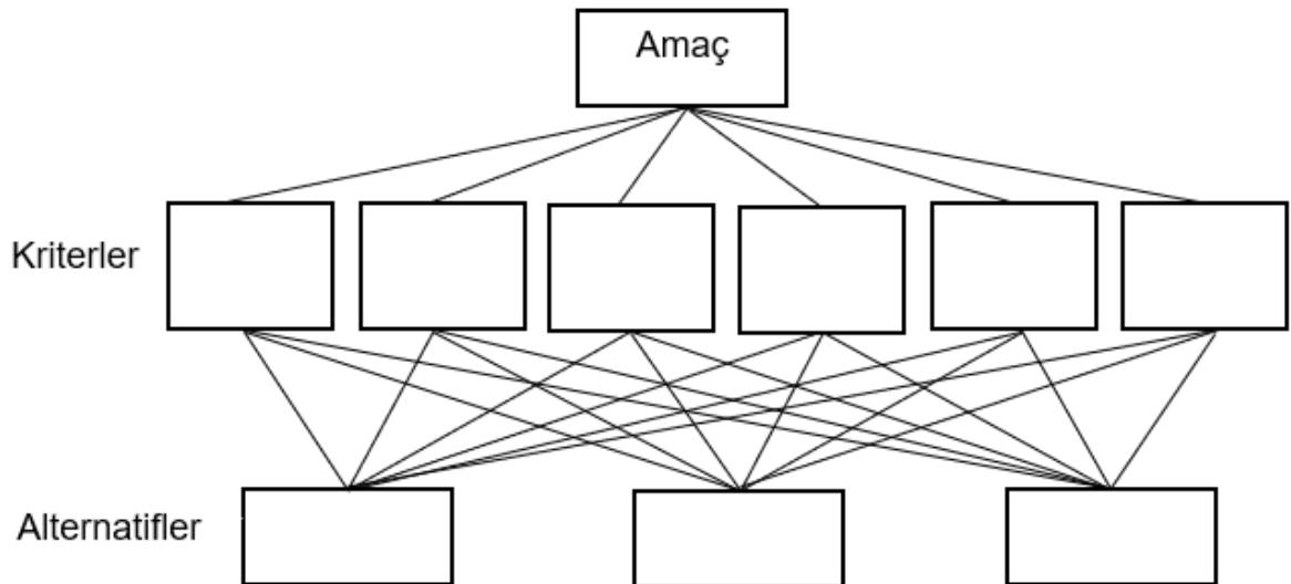
Şekil 3.1 Üç Seviyeli Analitik Hiyerarşi Modeli
