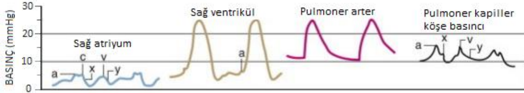
Şekil 2.4. Normal sağ kalp kateterizasyonu basınç örnekleri (56).
