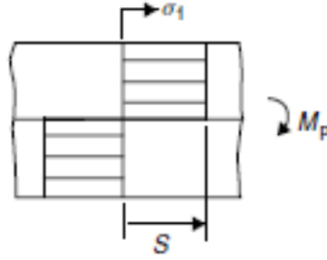
Şekil 4-6. Tamamen plastik bükmedeki gerilim dağılımı [21]
