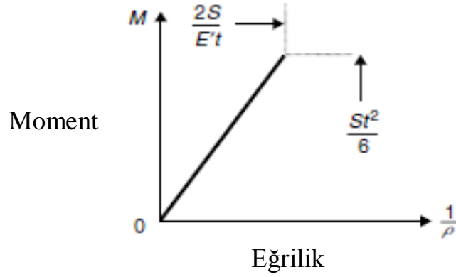
Şekil 4-7. Tamamen elastik bükmede oluşan moment-eğri grafiği [21]
