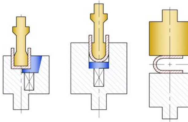
Şekil 4-13. U - Bükme İşleminin Süreçleri
